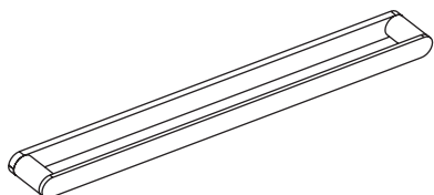
W: 24 3/4 D: 2 5/8 H: 1 1/4 2802 towel bar $290
